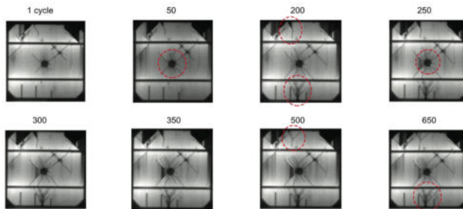
Figure 95: (ENG) Degradation of the electric response and increasing crack pattern at different bending cycles caused by fatigue. Taken from [358]. / (ESP) Degradación en la potencia eléctrica con el aumento de los ciclos de flexión a fatiga. Tomado de [358].
