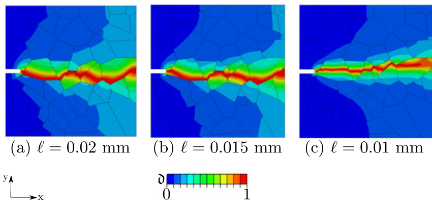
Figure 93: (ENG) Dependence of the crack propagation on the length scale \ell : results for a mesh refinement of h_e = 0.01\text{mm} / (ESP) Dependencia en la propagación de grieta del parámetro length scale \ell : resultados para una malla refinada de h_e = 0.01\text{mm} .
