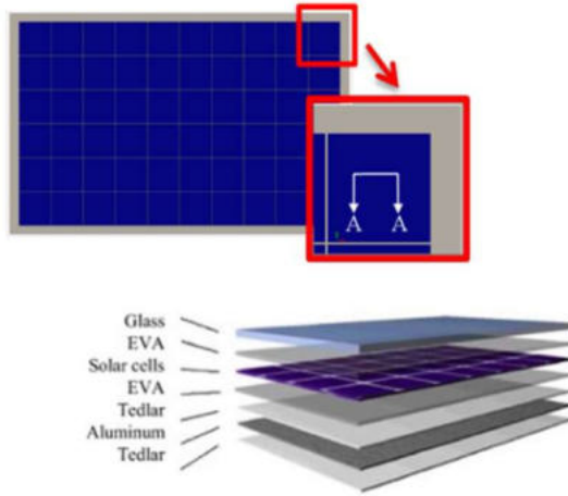
Figure 96: (ENG) Assembly of the laminate of a Si-based PV-module. / (ESP) Ensamblaje de un laminado de panel fotovoltaico de silicio.
