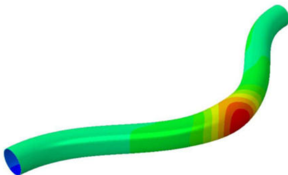
Figure 94: (ENG) Bulging instability occurring at the middle of a cylinder. Image taken from a numerical analysis from Desena-Galarza et al. [296]. / (ESP) Inestabilidad de hinchazón sucediendo en el medio de un cilindro. Imagen tomada de un análisis numérico llevado a cabo por Desena-Galarza et al. [296].
